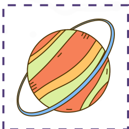
Uranus
